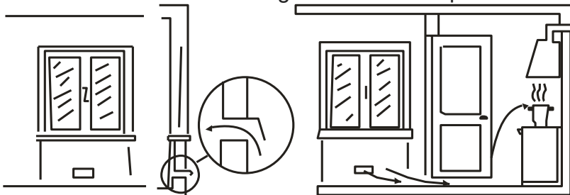
Detalles A: Habitación contigua - Habitación para ser ventilada
